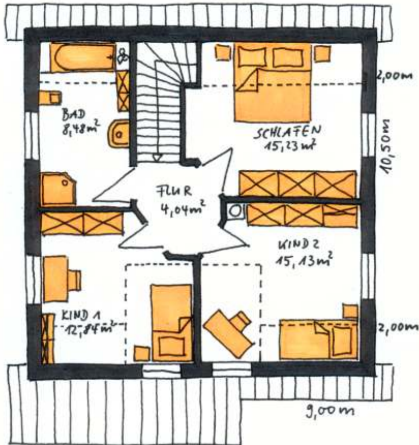
Obergeschoß Wohnfläche ca. 55,7m 2
