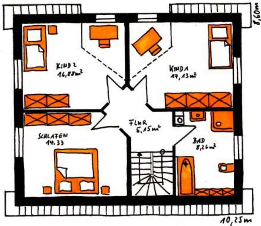
Obergeschoß Wohnfläche ca. 61,7m 2
