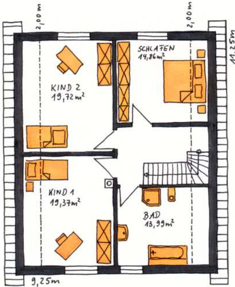
Obergeschoß Wohnfläche ca. 75,3m 2
