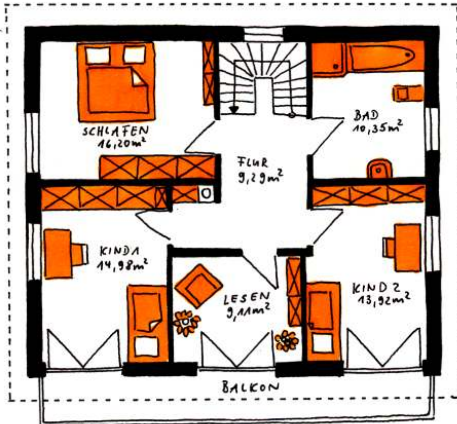
Obergeschoß Wohnfläche ca. 73,8m 2
